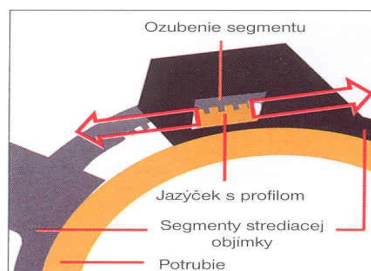
Obr. 2 Pričný rez
